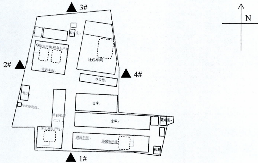
厂界环境噪声检测点位示意图 注：图中▲为厂界环境噪声检测点位
